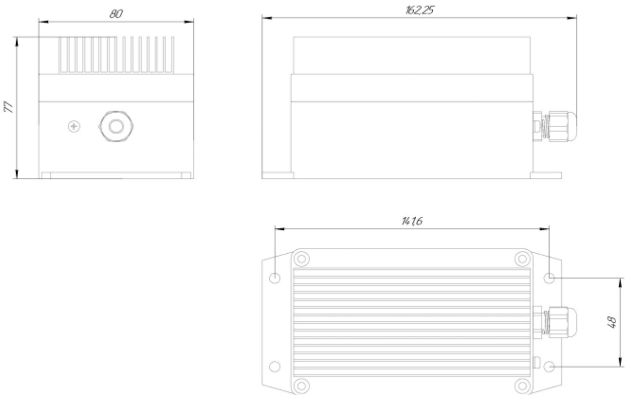
Рисунок А.2 – Габаритные размеры
